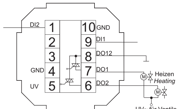
IO-Erweiterung Typ DO2T IO-Extension Type DO2T
