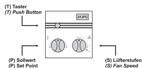
WRF04 LCD PST MODBUS AO2V
