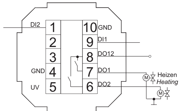
IO-Erweiterung Typ DO2R IO-Extension Type DO2R
