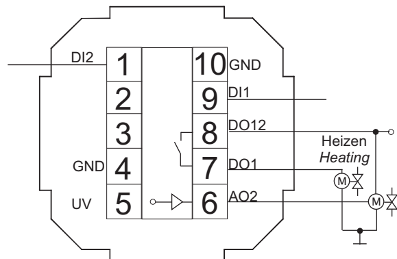
IO-Erweiterung Typ OVR IO-Extension Type OVR
