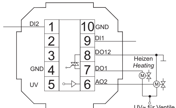
IO-Erweiterung Typ OVT IO-Extension Type OVT
