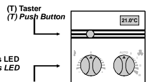
(T) Taster (T) Push Button (D) Status LED (D) Status LED (P) Sollwert (P) Set Point WRF04PST DSP
